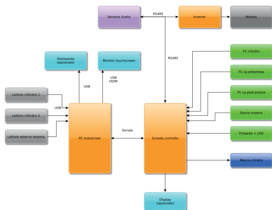
Sistema scheda elettronica - controllo macchine
